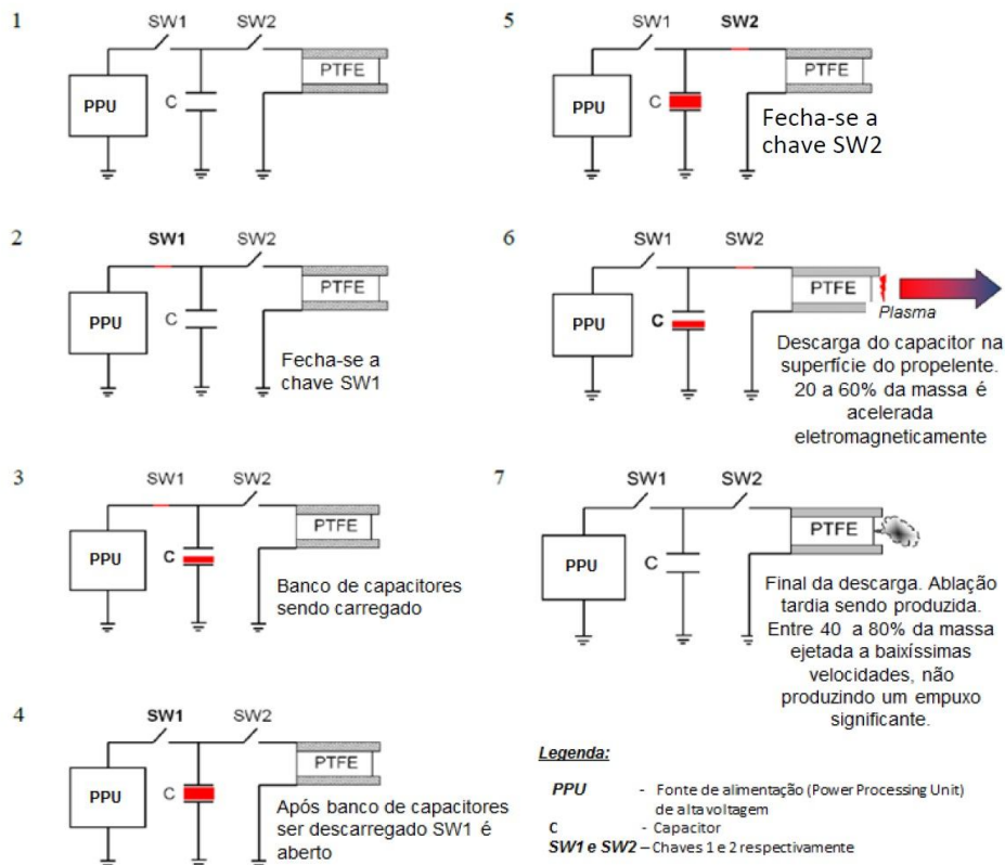
Figura 2: Mecanismo de carga e descarga de um ppt básico fonte: Intini Marques (2009) adaptado por MARIN (2014)
