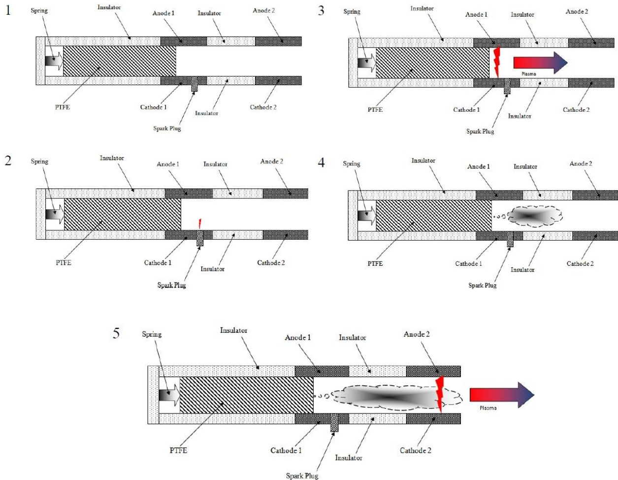
Figura 3: esquema da seqüência de descarga do TS-PPT Fonte: Intini Marques (2009)
