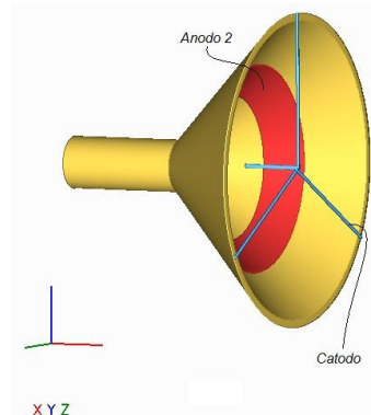
Figura 5: Geometria da proposta de um PPT cônico
