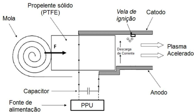
Figura 1: Diagrama básico de um propulsor de plasma pulsado fonte: Intini Marques (2009) adaptado por MARIN (2014)
